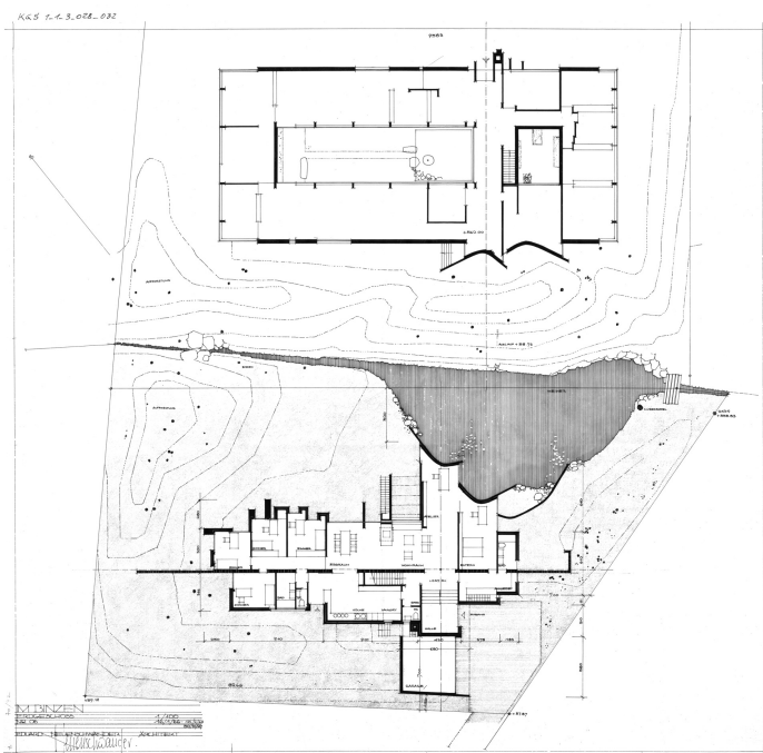
Wohnhaus Im Binzen, Grundrissplan, oben Atelier Neuenschwander (Vers. Nr. 02454, 04340), unten Wohnhaus Im Binzen (Vers. Nr. 02943), Baueingabeplan 16.01.1966, Bild: Planarchiv kantonale Denkmalpflege Zürich (Bild Nr. P1_1_3_028_032).
